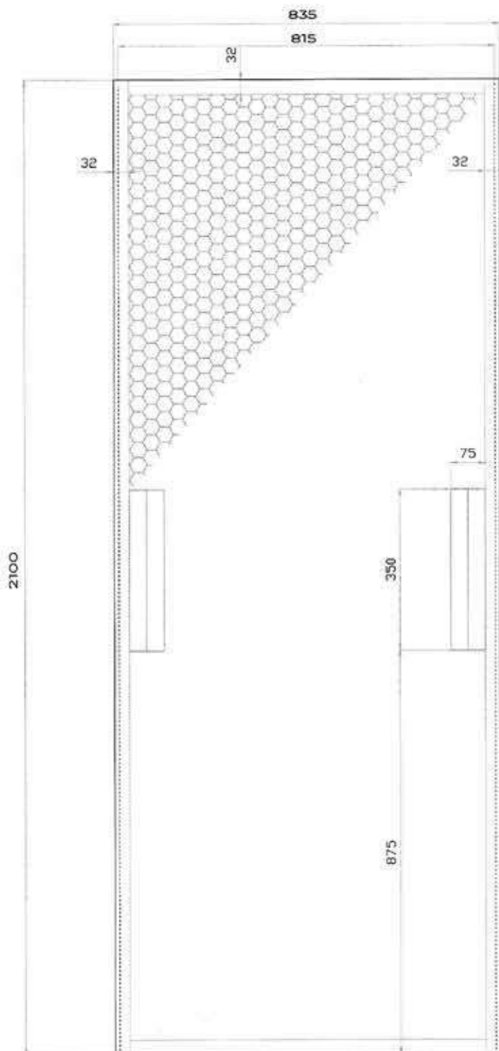
PROSPETTO ANTA
