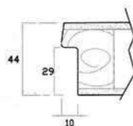
SEZIONE VERTICALE
