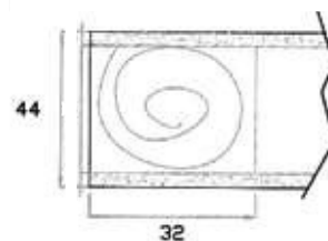
SEZIONE VERTICALE
